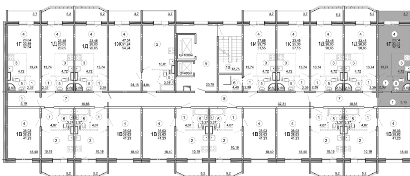
План этажа:
