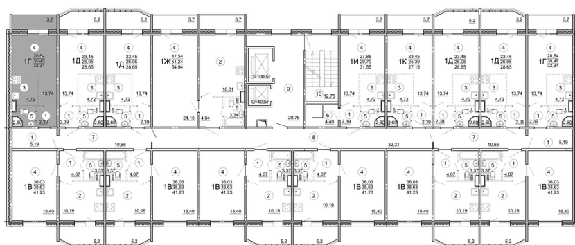
План этажа:
