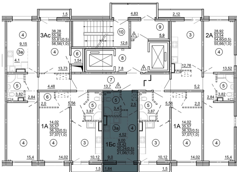
План этажа:
